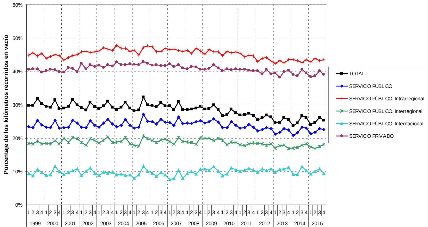
EVOLUCIÓN DE LA ACTIVIDAD SEGÚN EL TIPO DE SERVICIO Y DESPLAZAMIENTO VEHÍCULOS PESADOS y recorridos intermunicipales Porcentaje de los kilómetros recorridos en vacío sobre el total de kilómetros recorridos
