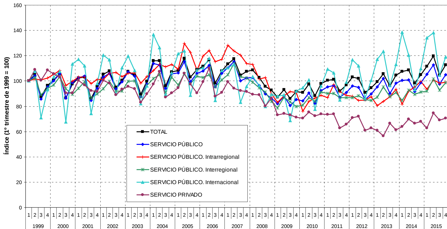
EVOLUCIÓN DE LA ACTIVIDAD SEGÚN EL TIPO DE SERVICIO Y DESPLAZAMIENTO VEHÍCULOS PESADOS y recorridos intermunicipales Toneladas-kilómetro producidas / Toneladas ofertadas
