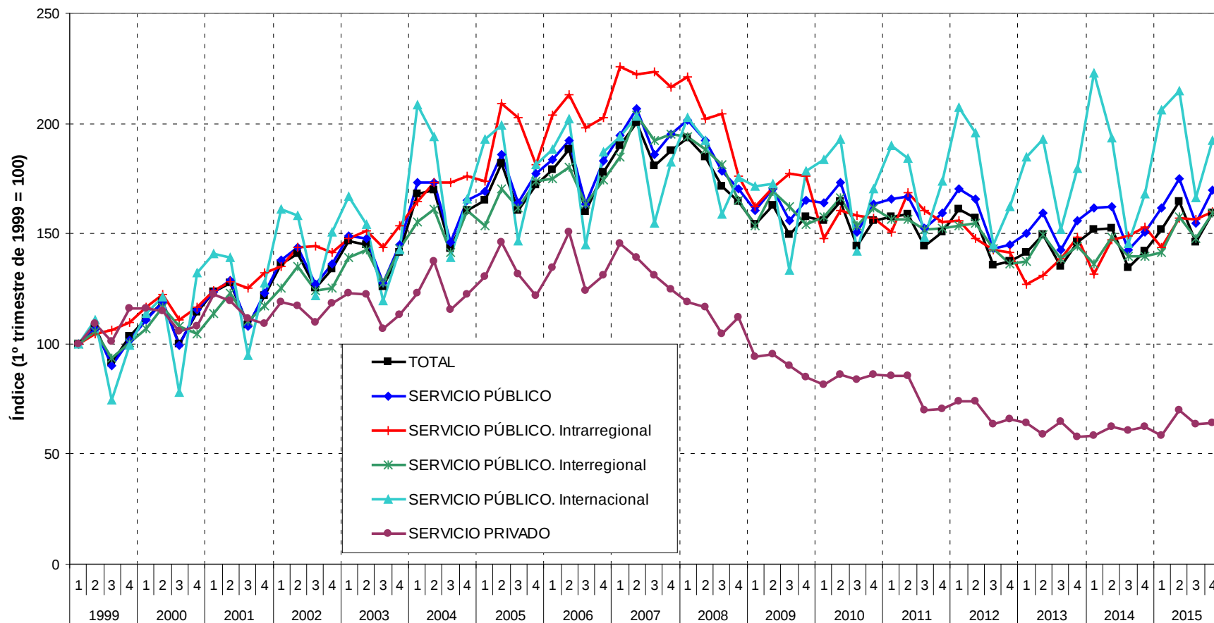
EVOLUCIÓN DE LA ACTIVIDAD SEGÚN EL TIPO DE SERVICIO Y DESPLAZAMIENTO VEHÍCULOS PESADOS y recorridos intermunicipales Toneladas-kilómetro producidas
